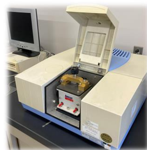
フーリエ変換型赤外分光光度計 (株)島津製作所製 IR Prestige-21
